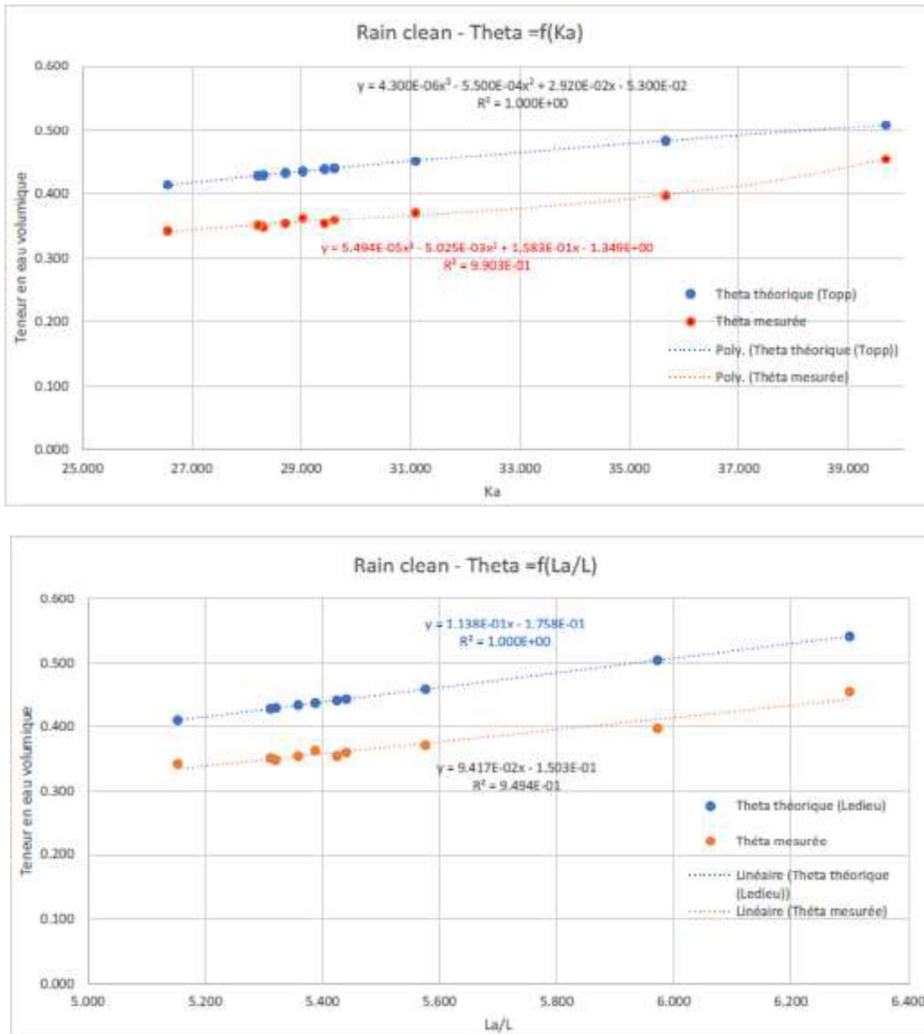
Figure 5 : courbe de calibration des sondes pour le rainclean.
