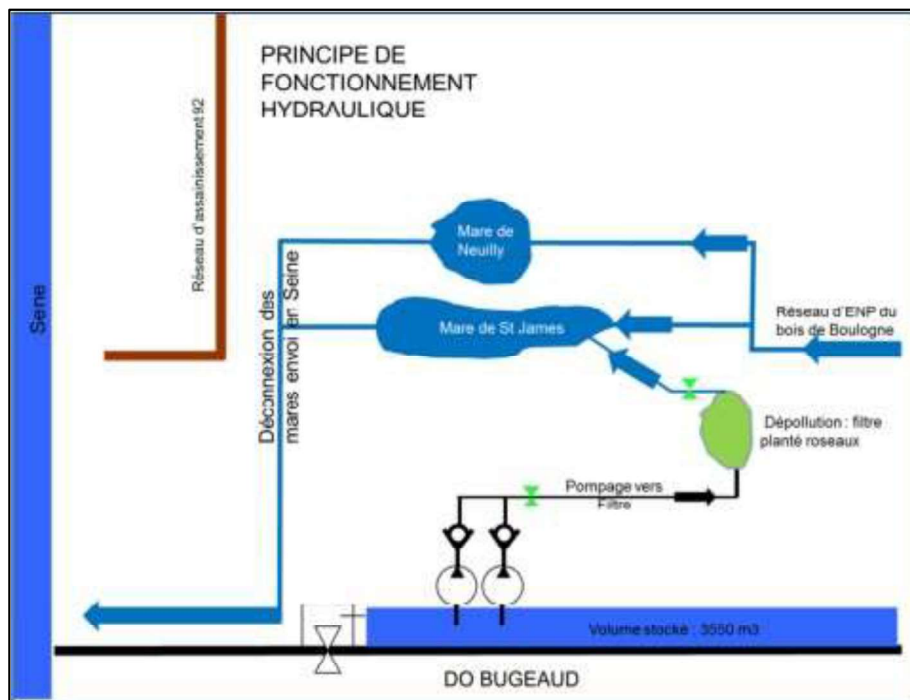
Figure 1 : schéma de principe du système étudié.
