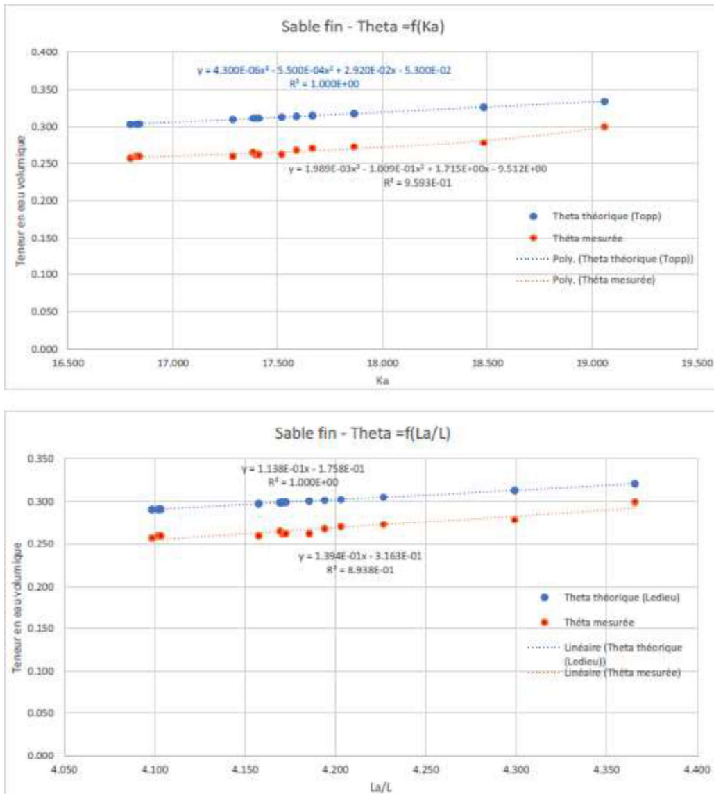
Figure 4 : courbe de calibration des sondes pour le sable fin.
